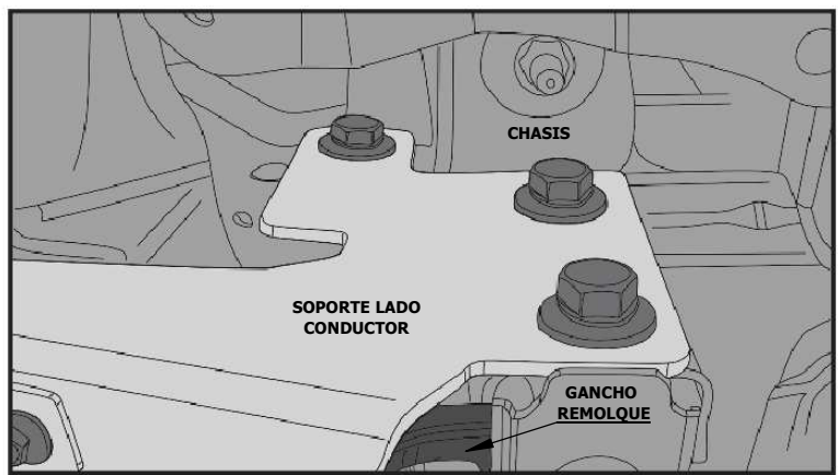
SOPORTE VISTA INFERIOR LADO CONDUCTOR
